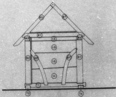
KELETI HOMLOKZAT
