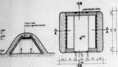
ALAPRAJZ
