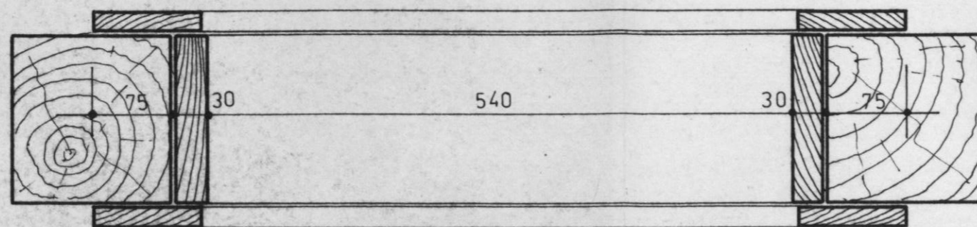
KERESZTMETSZET
